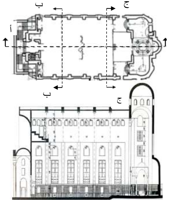
قطاع رأسى طولى أ-أ بجسم الكنيسة
