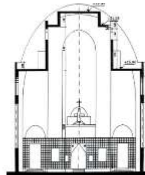
قطاع رأسى عرضى ب-ب وبه الضلع الشرقي
