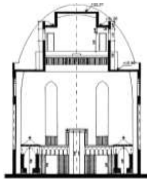
قطاع رأسى عرضى ج-ج وبه الضلع الغربي
